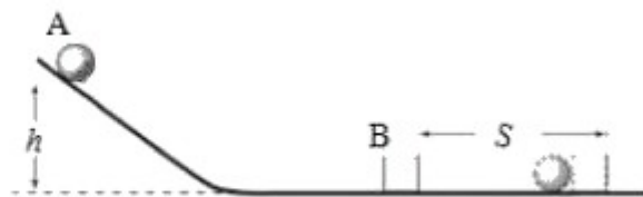
乙 探究物体动能与哪些因素有关
